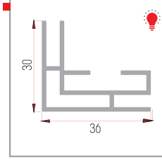
30 mm (0,607 kg/m)
