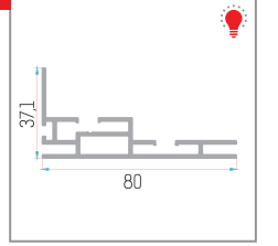
80 mm (0,9 kg/m)
