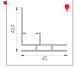
45 mm (0,626 kg/m)
