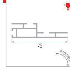
75 mm (0,986 kg/m)
