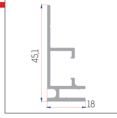
18 mm (0,412 kg/m)
