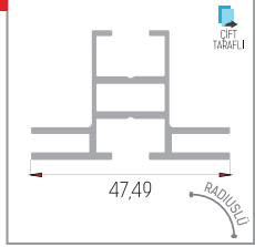
47 mm (0,688 kg/m)
