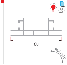
60 mm (0,845 kg/m)
